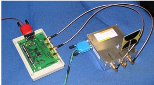
Fig. 2. UWB pulse generator.
